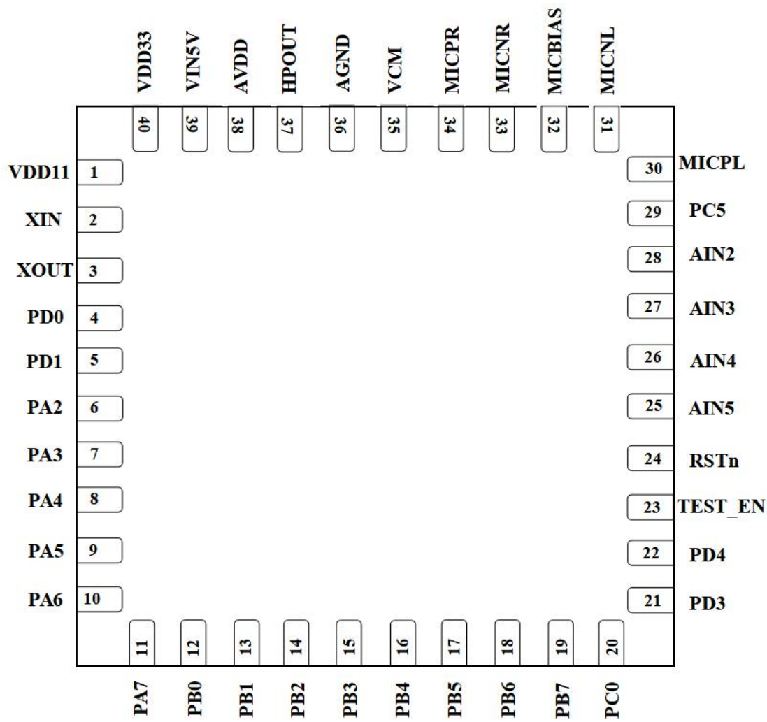
图 2: QFN40 引脚图
