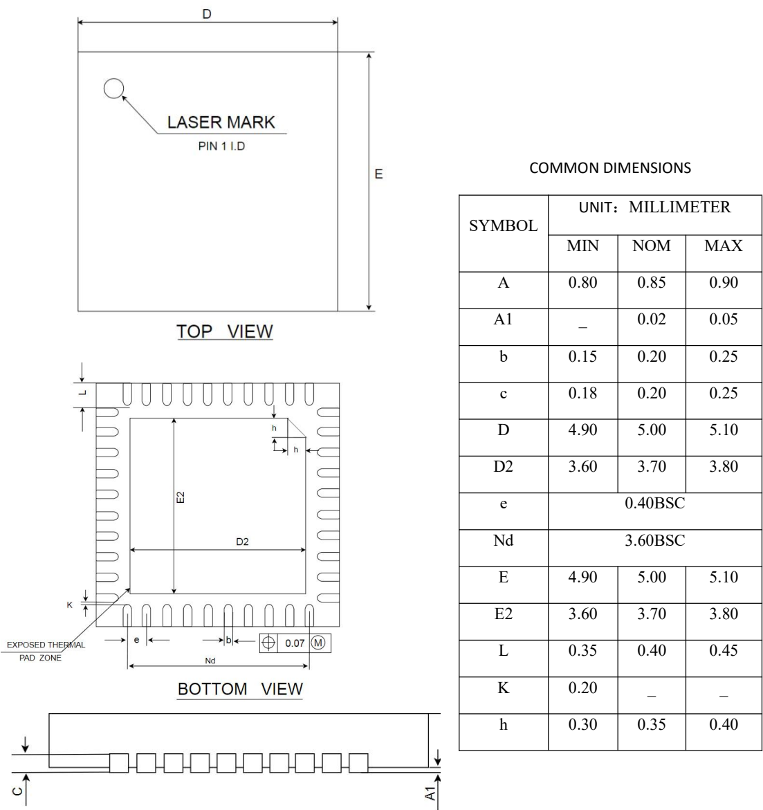
图 10：封装尺寸
